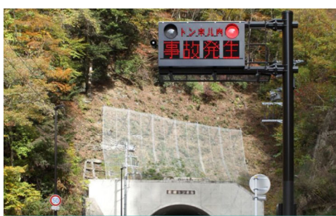
トンネル非常警報設備設計
