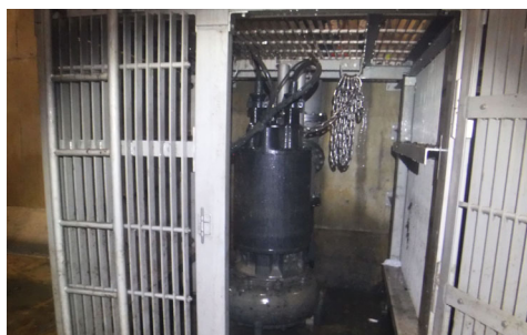
ポンプ用電気設備設計
